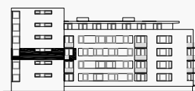
Severní pohled
